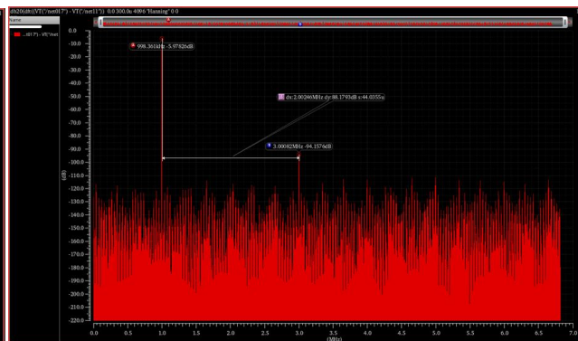
图表 10 THD5V
