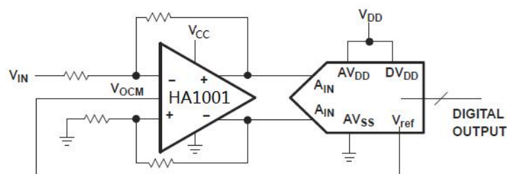
图 1 HA1001E 典型应用图
