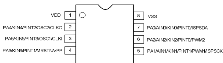
SOP8 顶视图
