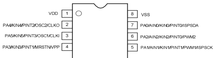
DFN8 顶视图
