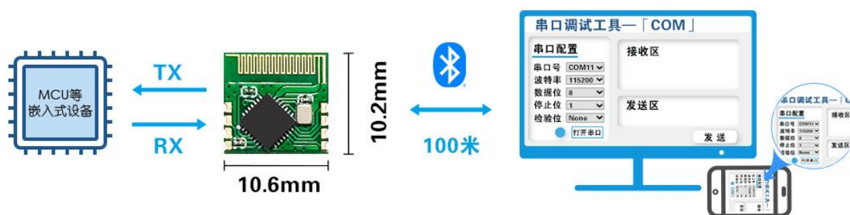
图 1 蓝牙主机通过 CH9140 蓝牙与串口设备进行串口通讯框图
