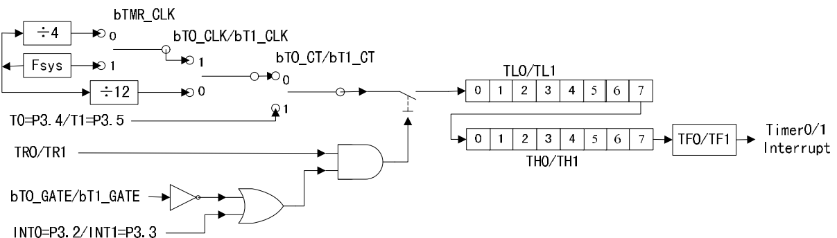
图 12.5.1.2 Timer0/1 模式 1
