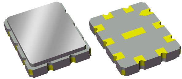
SMP-35B, 9.0 x 7.01 x 1.50 mm
