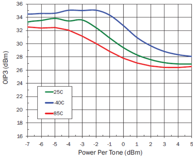
OIP3 versus Power Out ( V_D = 5\text{V} , 900MHz)
