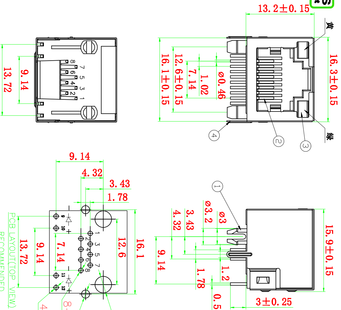
网络插座外形图
