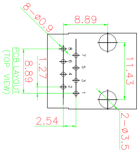
网络插座外形图
