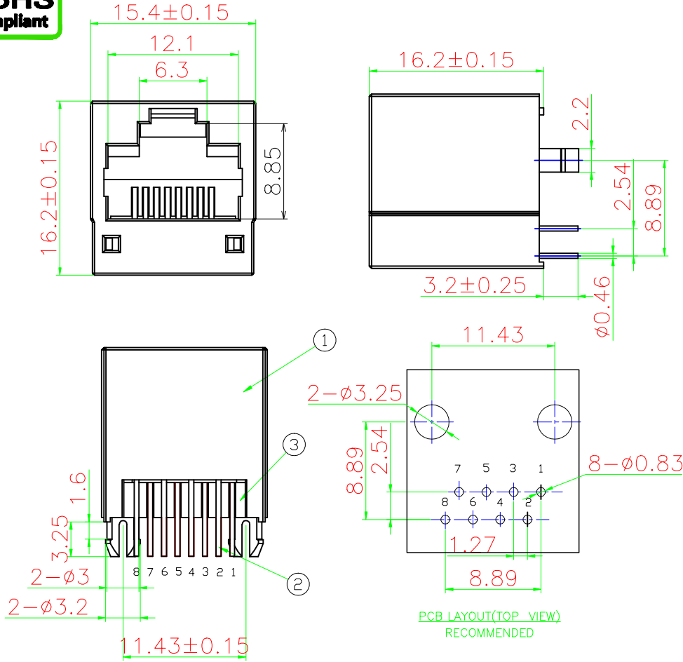
网络插座外形图
