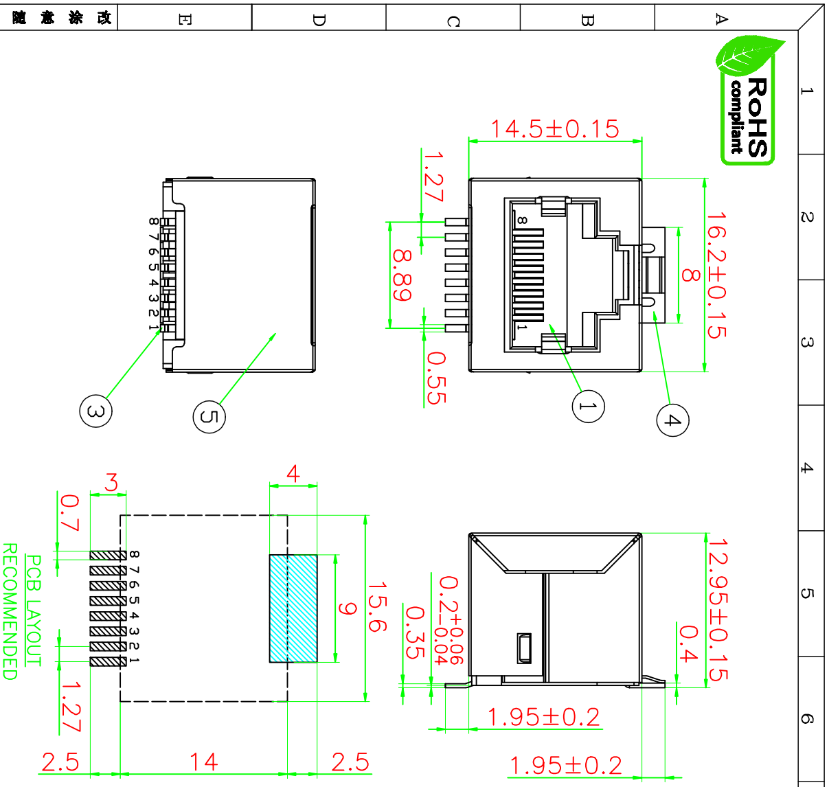
网络插座外形图
