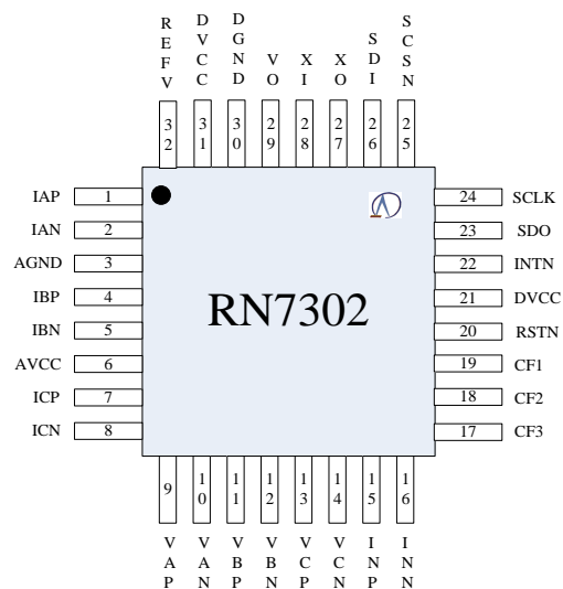
图 2-2 管脚排列图
