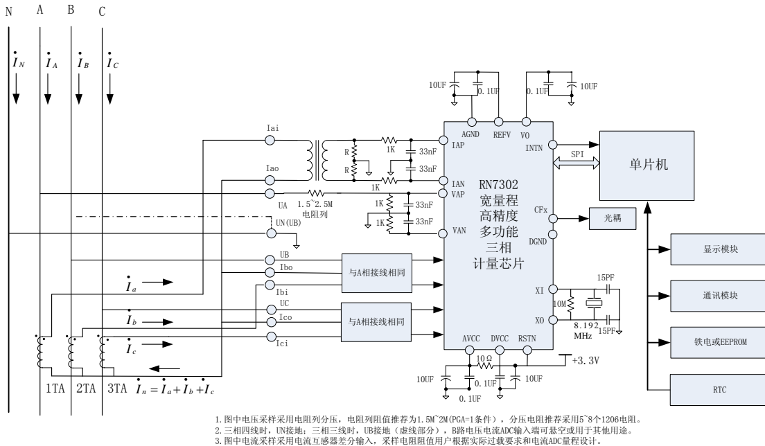
图 1-3 典型应用电路示意图 1
