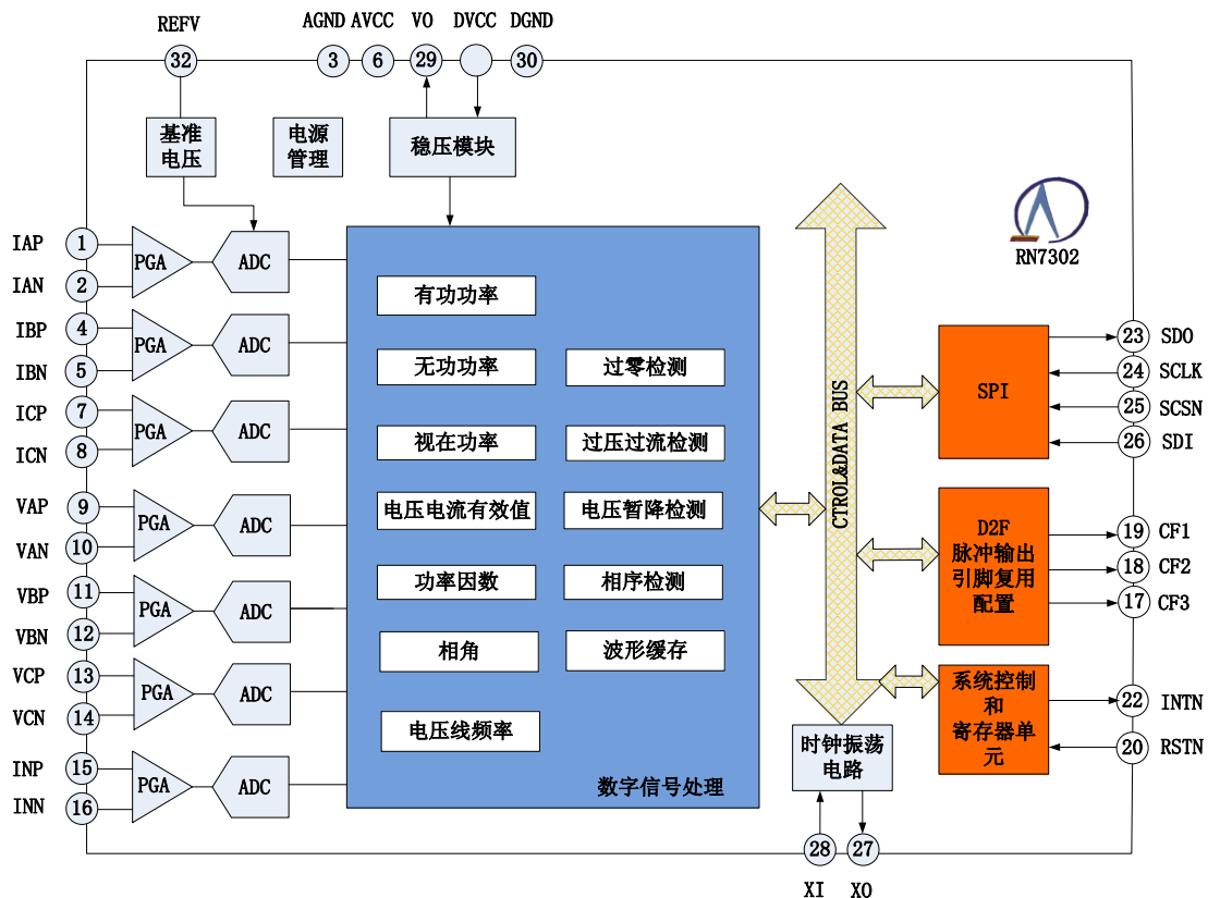
图 2-1 系统框图
