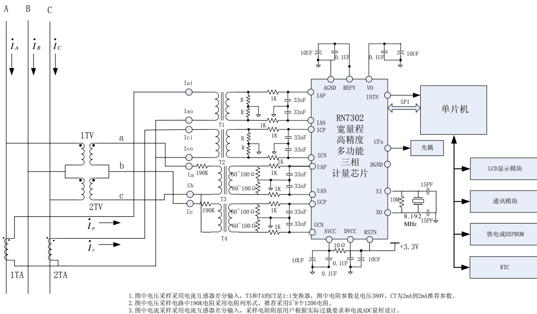
图 1-4 典型应用电路示意图 2
