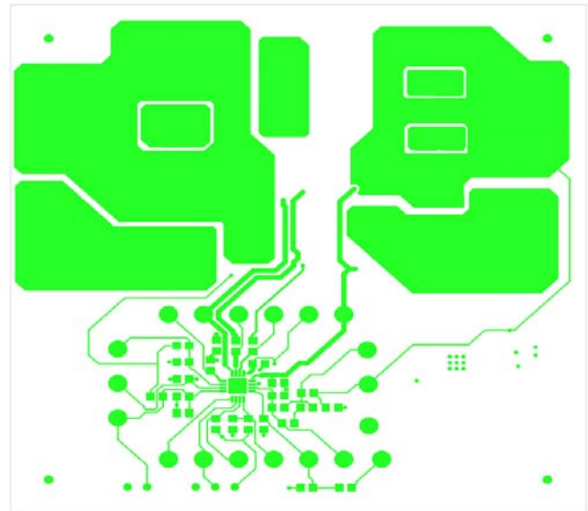
FIGURE 22. TOP LAYER
