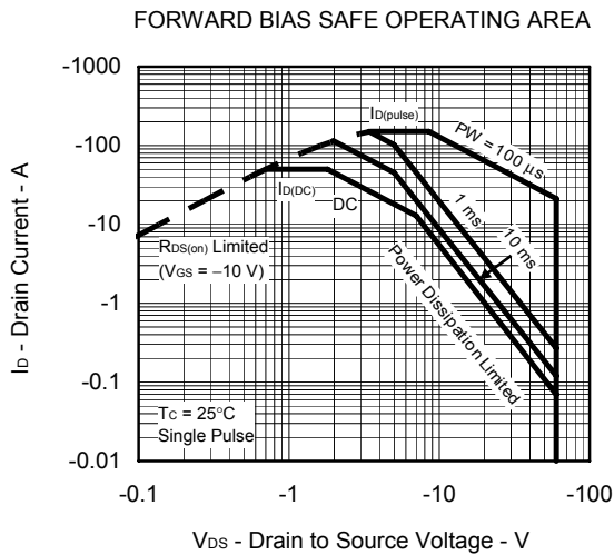
V DS - Drain to Source Voltage - V
