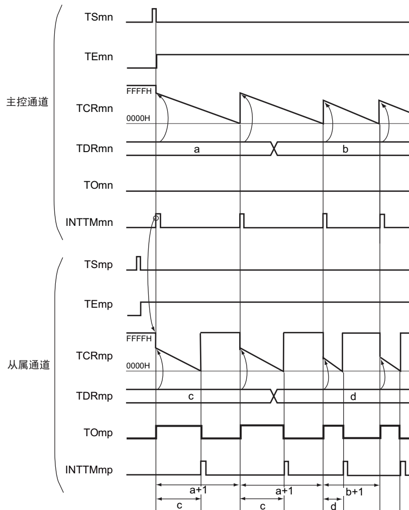
图 6-73 作为 PWM 功能的运行基本时序例子
