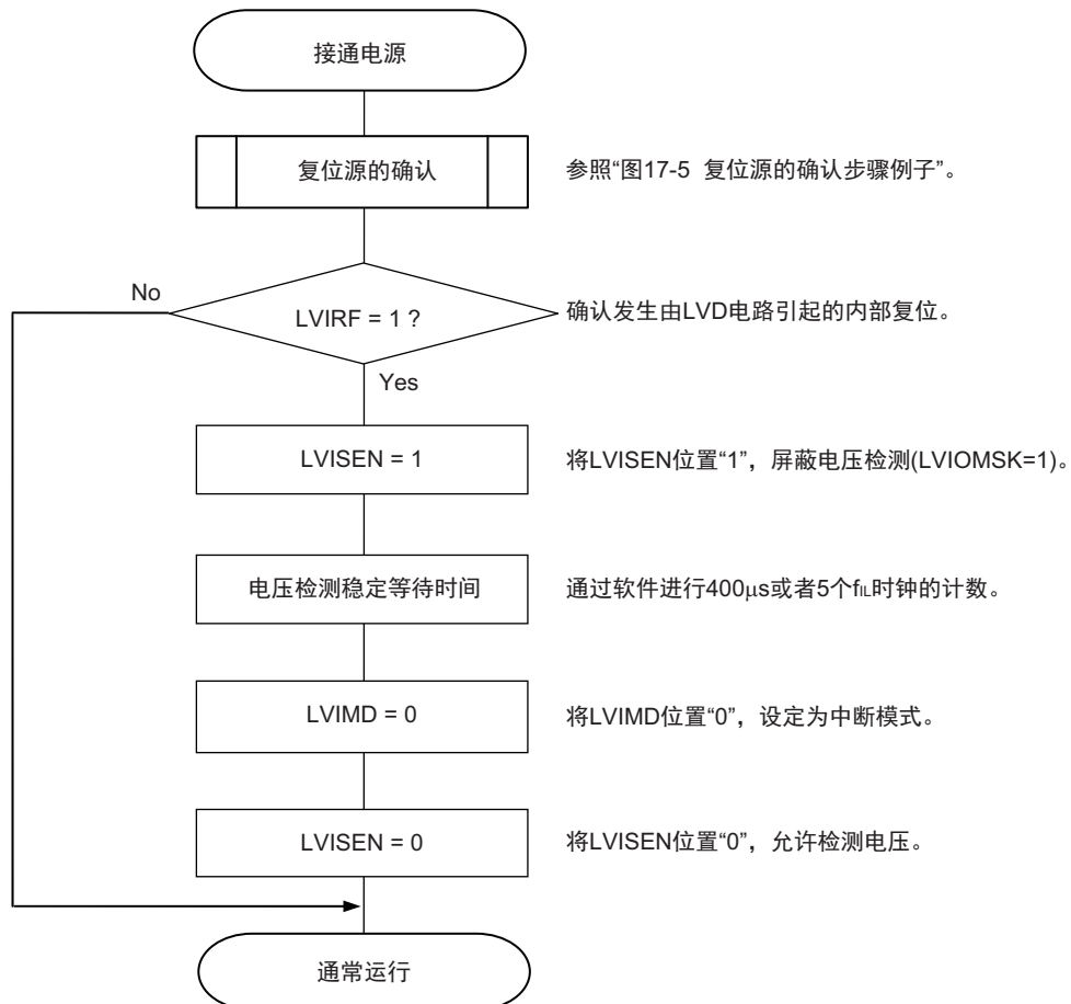
图 19-9 中断 & 复位模式的初始设定步骤
