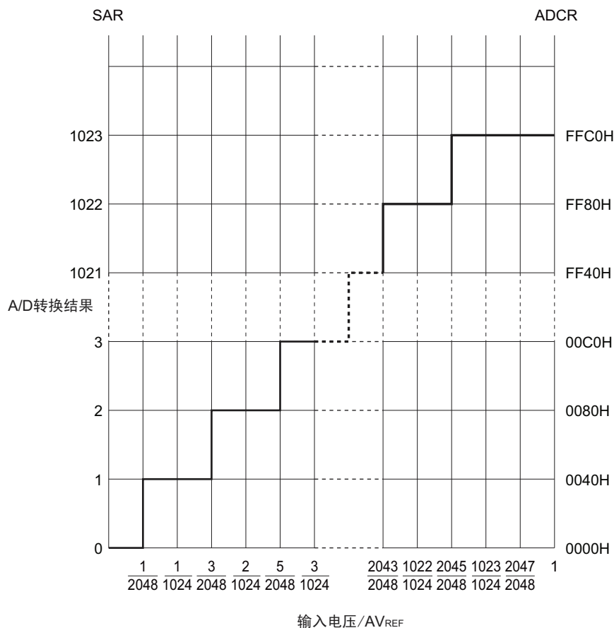
图 11-16 模拟输入电压和 A/D 转换结果的关系
