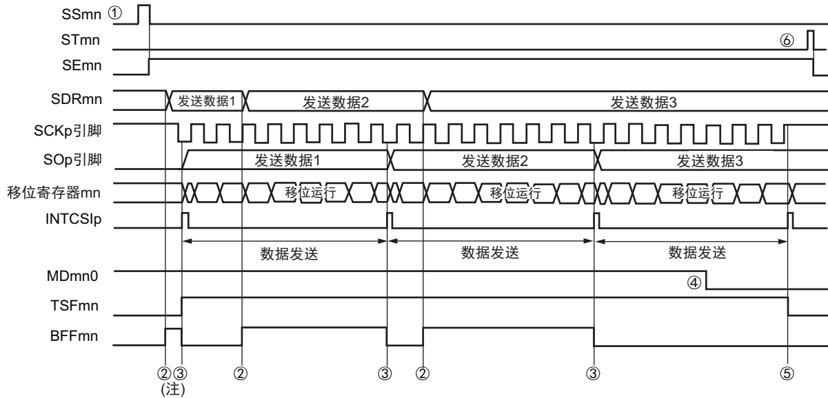
图 12-52 从属发送（连续发送模式）的时序图（类型 1：DAPmn=0、CKPmn=0）
