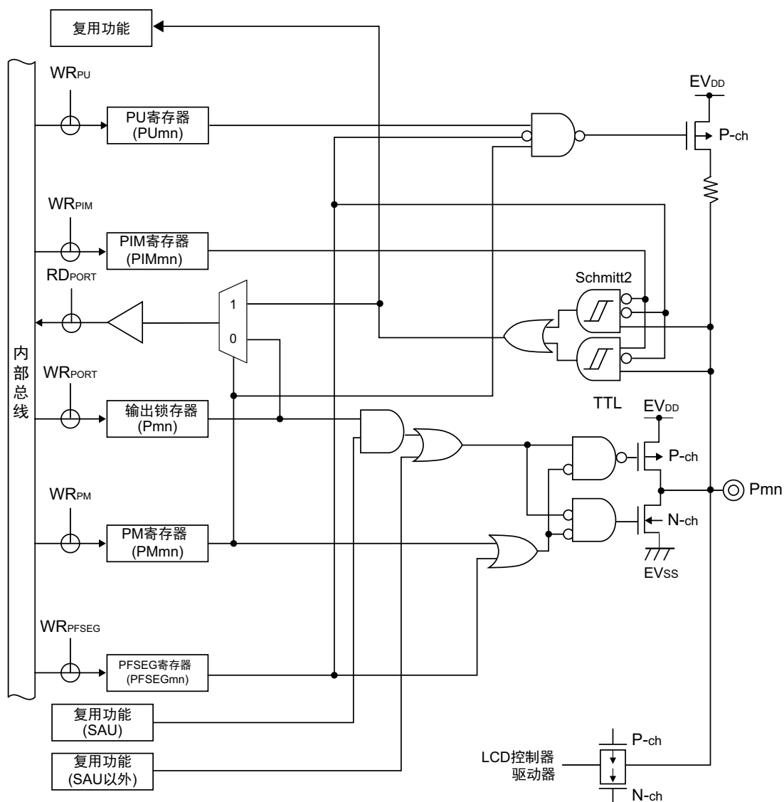
图 2-10 引脚类型 8-5-1 的引脚框图
