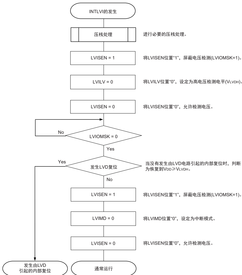
图 19-8 工作电压的确认 / 复位的设定步骤
