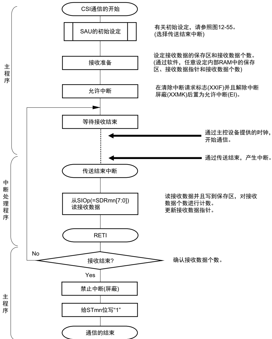
图 12-59 从属接收（单次接收模式）的流程图
