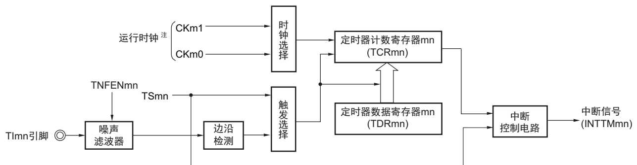
图 6-63 作为延迟计数器运行的框图
