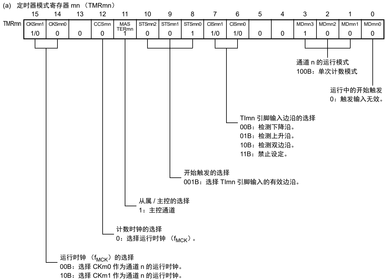
图 6-69 单触发脉冲输出功能时（主控通道）的寄存器设定内容例子
