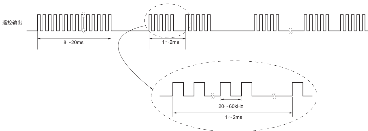
图 6-82 遥控输出
