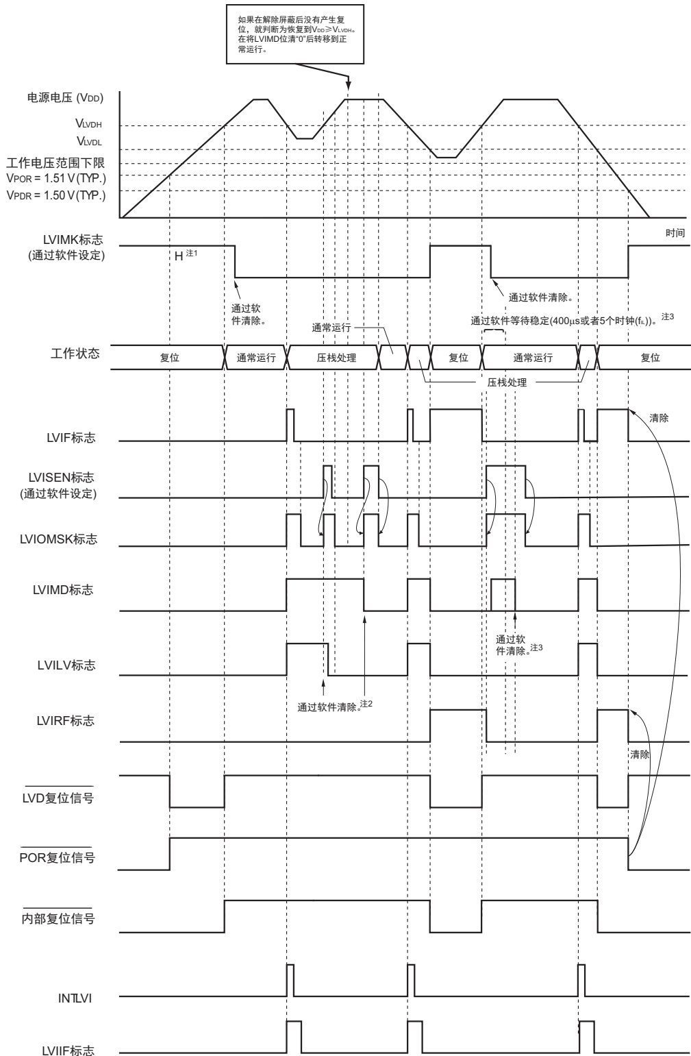
图 19-7 复位 &amp; 中断信号的发生时序 (选项字节的 LVIMDS1、LVIMDS0=1、0) (1/2)
