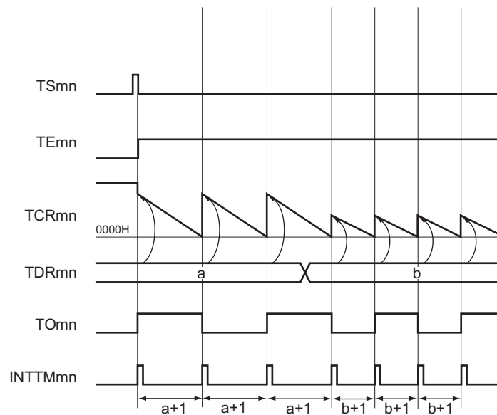
图 6-44 作为间隔定时器 / 方波输出运行的基本时序例子 (MDmn=1)
