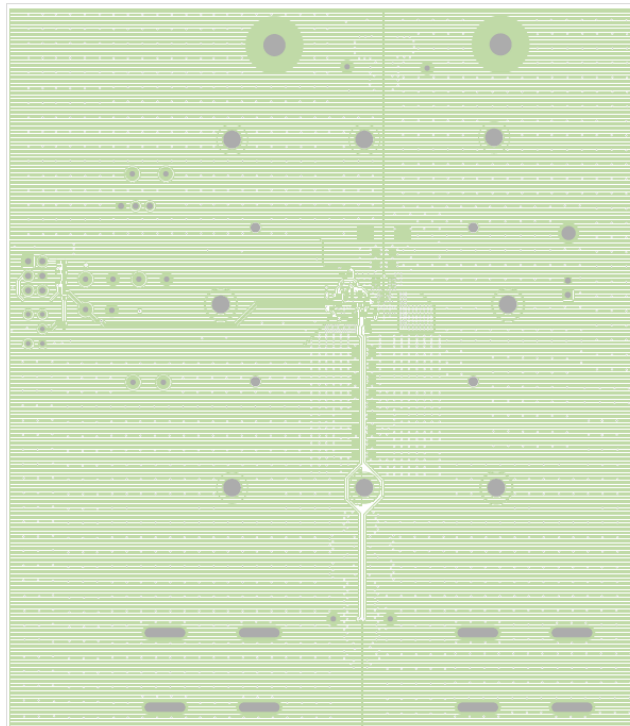
Figure 20. Bottom Layer
