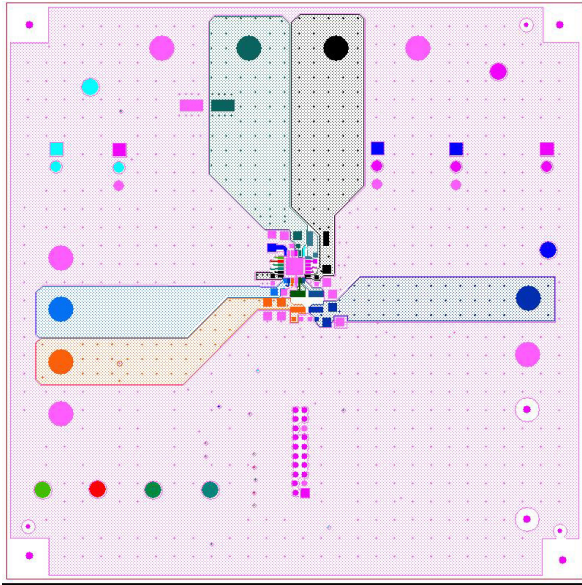
Figure 22. Top Layer
