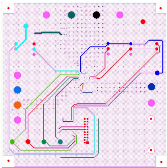
Figure 24. Layer 3
