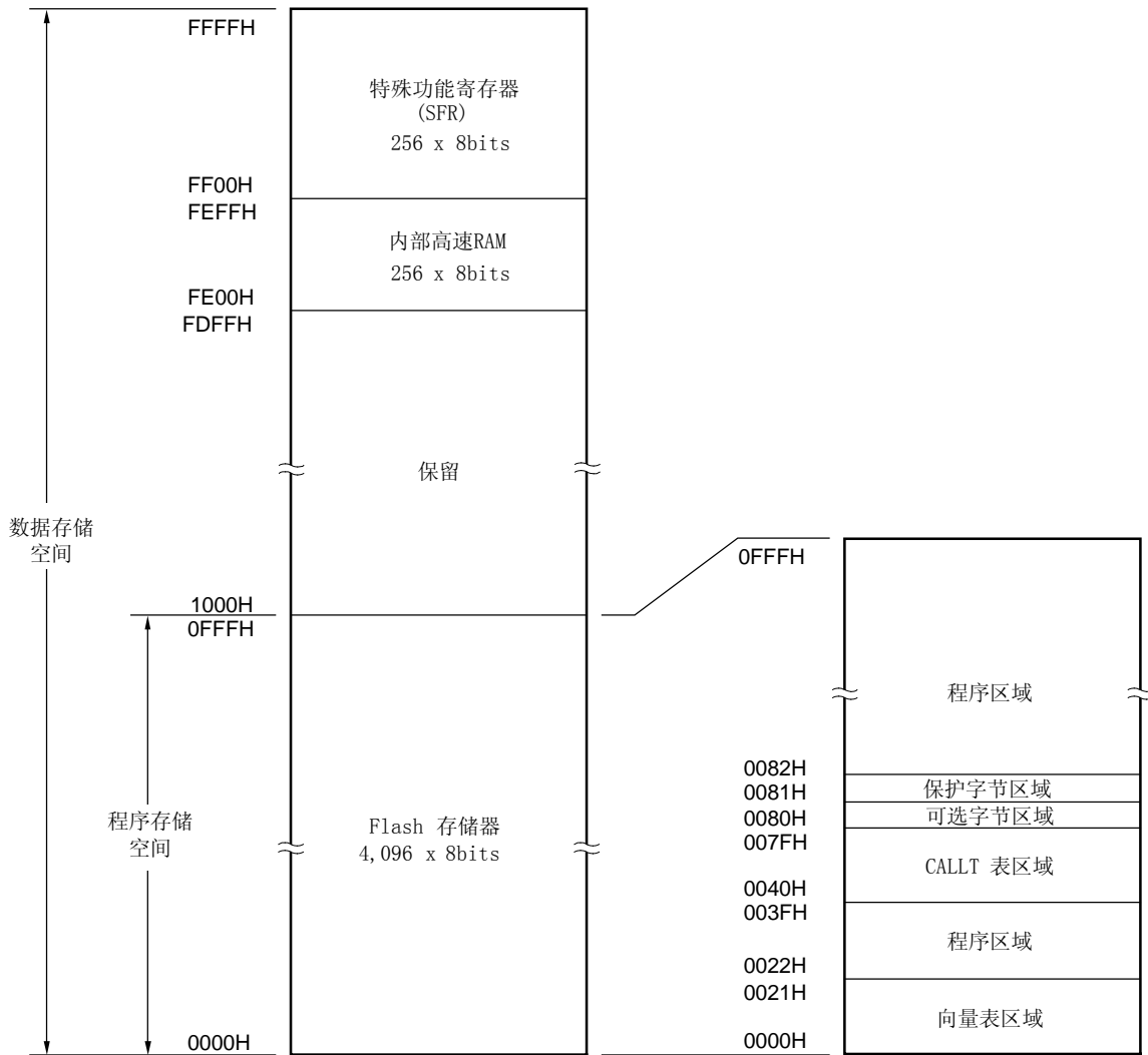
图 3-1. 存储空间映射图 ( \mu PD78F9232)
