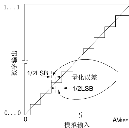
图 10-14. 总误差
