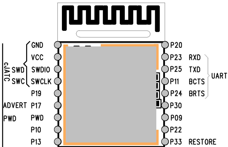
图 3 模块引脚定义图
