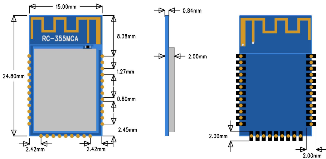
图2 模块尺寸图
