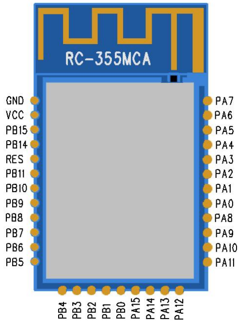
图 3 模块引脚定义图
