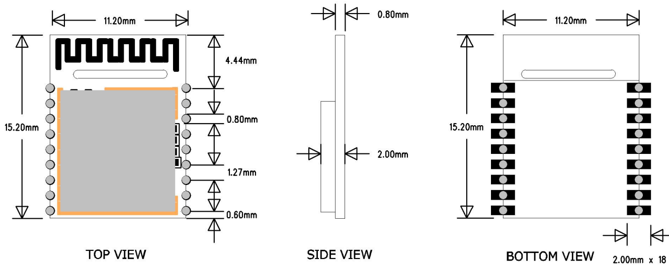
图2 模块尺寸图
