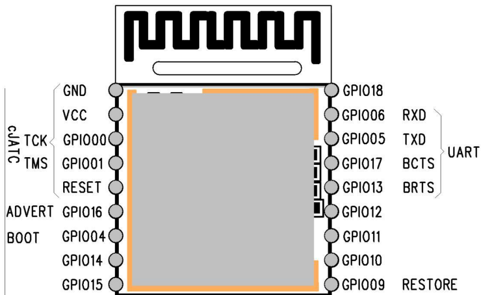
图3 模块引脚定义图
