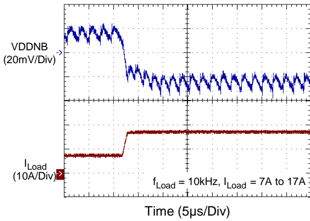
NB VR Load Transient
