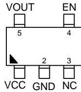
SOT-23-5
