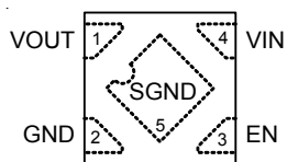
ZQFN-4L 1x1 (ZDFN-4L 1x1)
