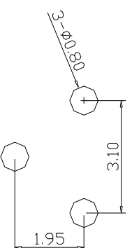
PCB. 焊接图
