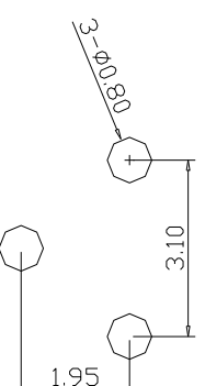
PCB. 焊接图
