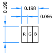
DETAIL A 60:1
