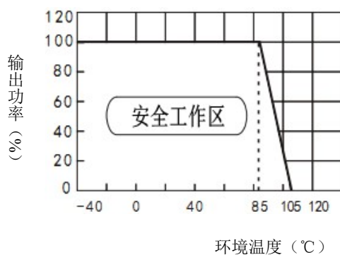
温度曲线图
