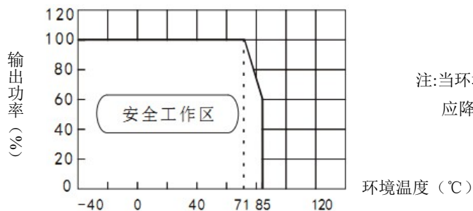
温度曲线图
