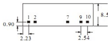
底视图
