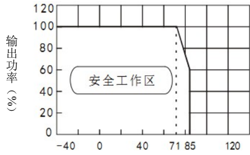
温度曲线图
