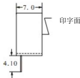
侧视图
