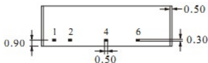
底视图
