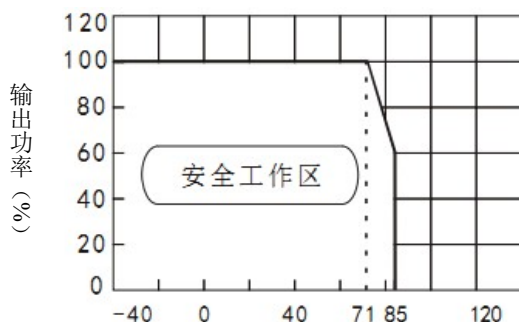
温度曲线图
