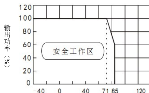
温度曲线图
