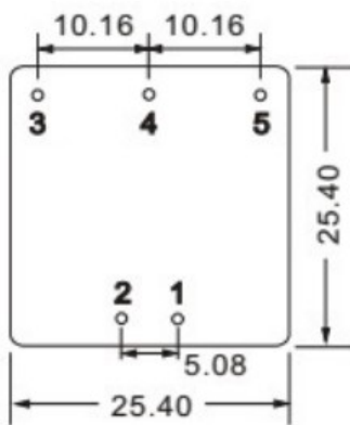
底视图
