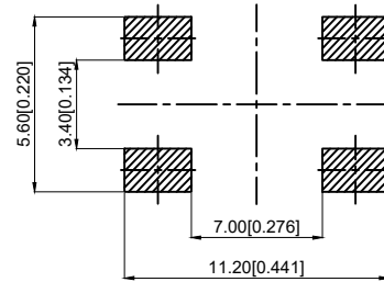
PCB LAND DIMENSION PCB电路板焊盘尺寸
