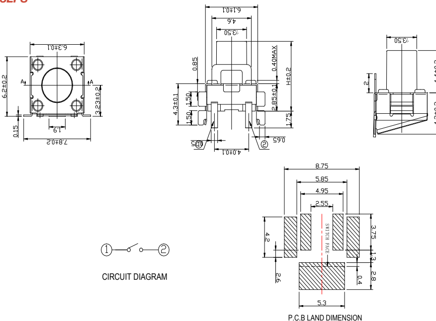
P.C.B. LAND DIMENSION
