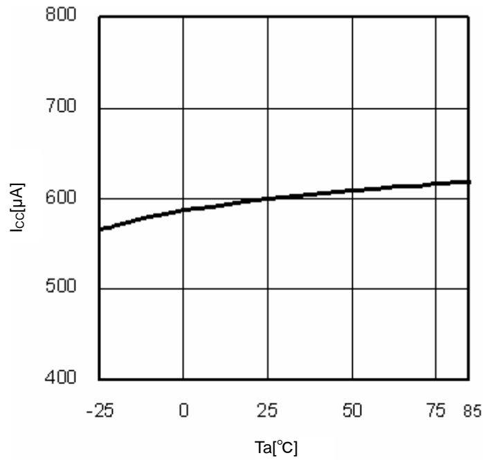
Fig.9 Ta-I cc
