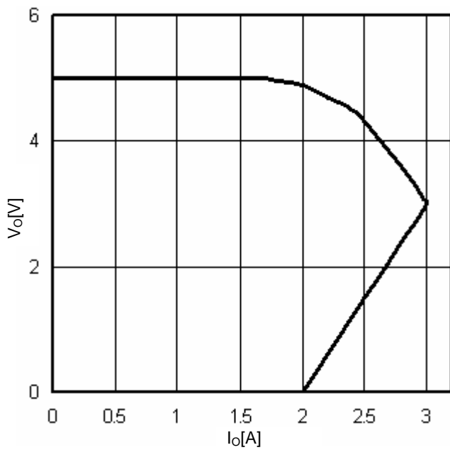
Fig.16 OCP
