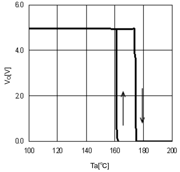
Figure 28. TSD ( I_o=0\text{mA} )
