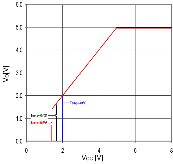
Fig.27 Vcc-Vo (Io=0mA)
