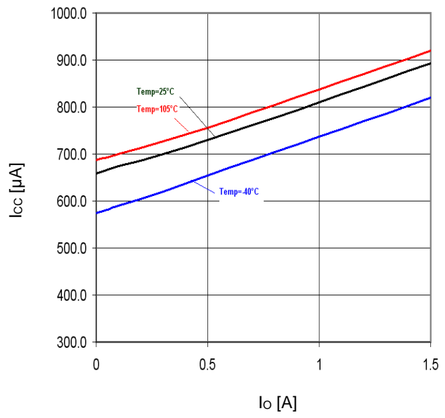
Fig.32 Io-Icc
