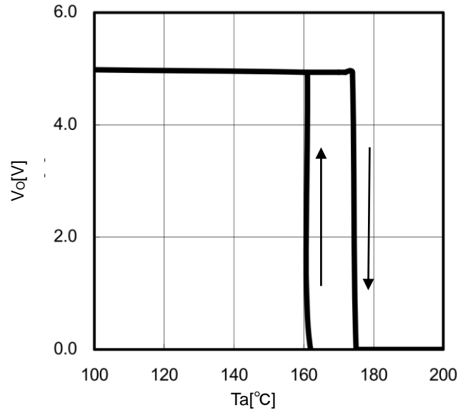
Fig.28 TSD (Io=0mA)
