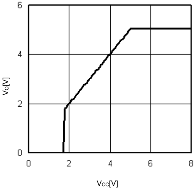
Fig.15 V_{cc}-V_o ( I_o=0\text{mA} )
