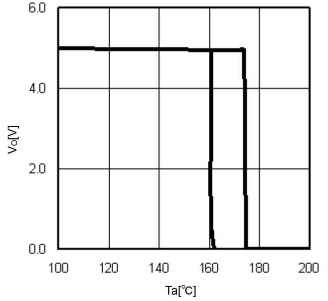
Fig.16 TSD ( I_o=0\text{mA} )
