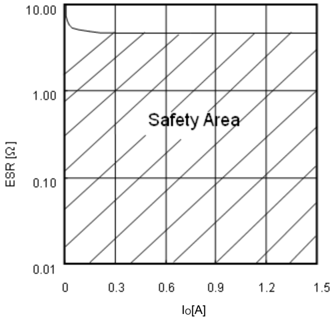
Fig.19 ESR condenser
