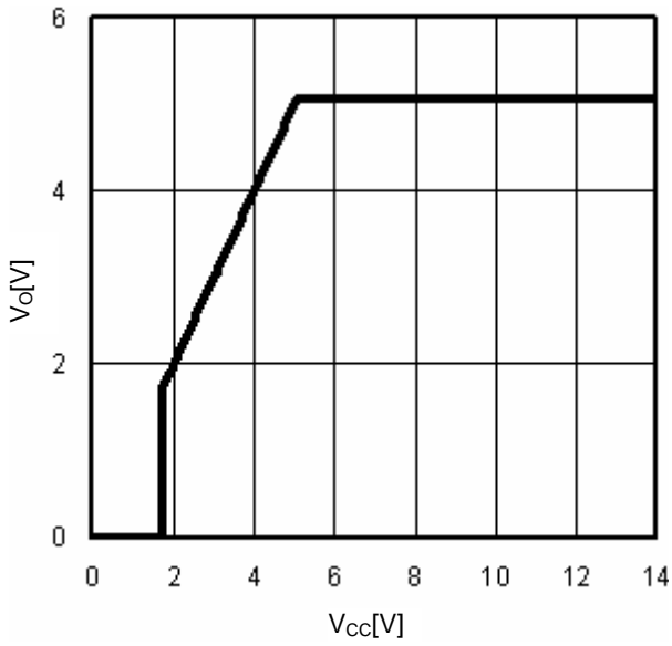
Fig.15 V_{cc}-V_o ( I_o=0mA )
