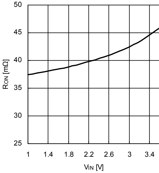
Figure.7 VIN-ROn
