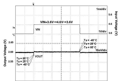
Fig 154. VIN Response
