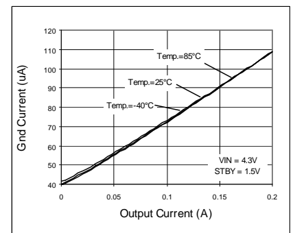
Fig. 16 IOUT - IGDND
