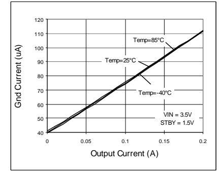
Fig. 71 IOU - IGND
