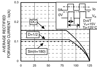
AMBIENT TEMPERATURE : T_a (°C) Derating Curve*( I_o - T_a )
