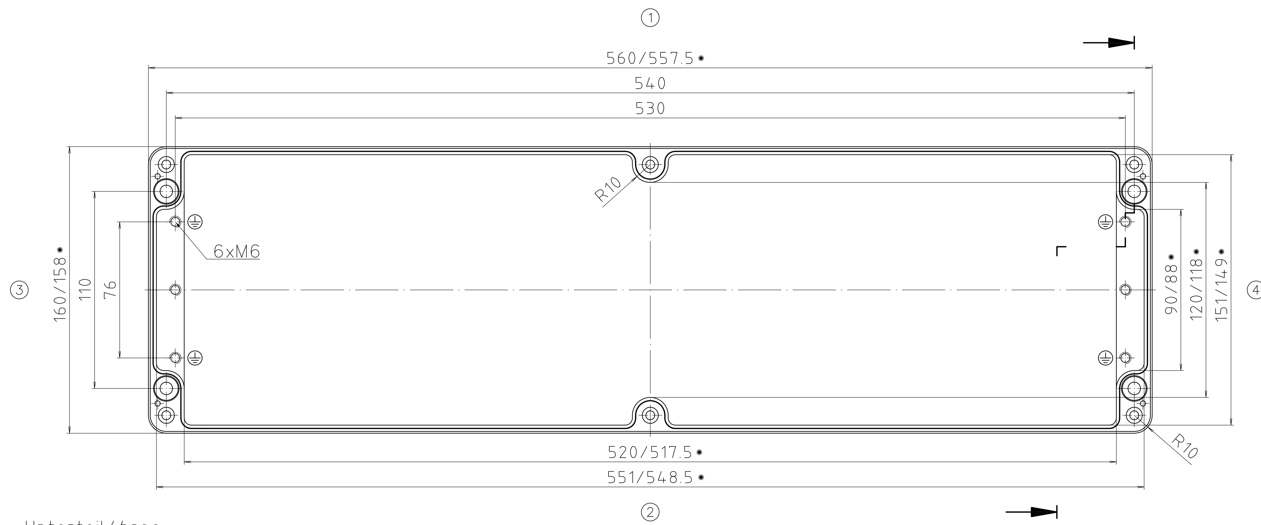
Unterteil / base
