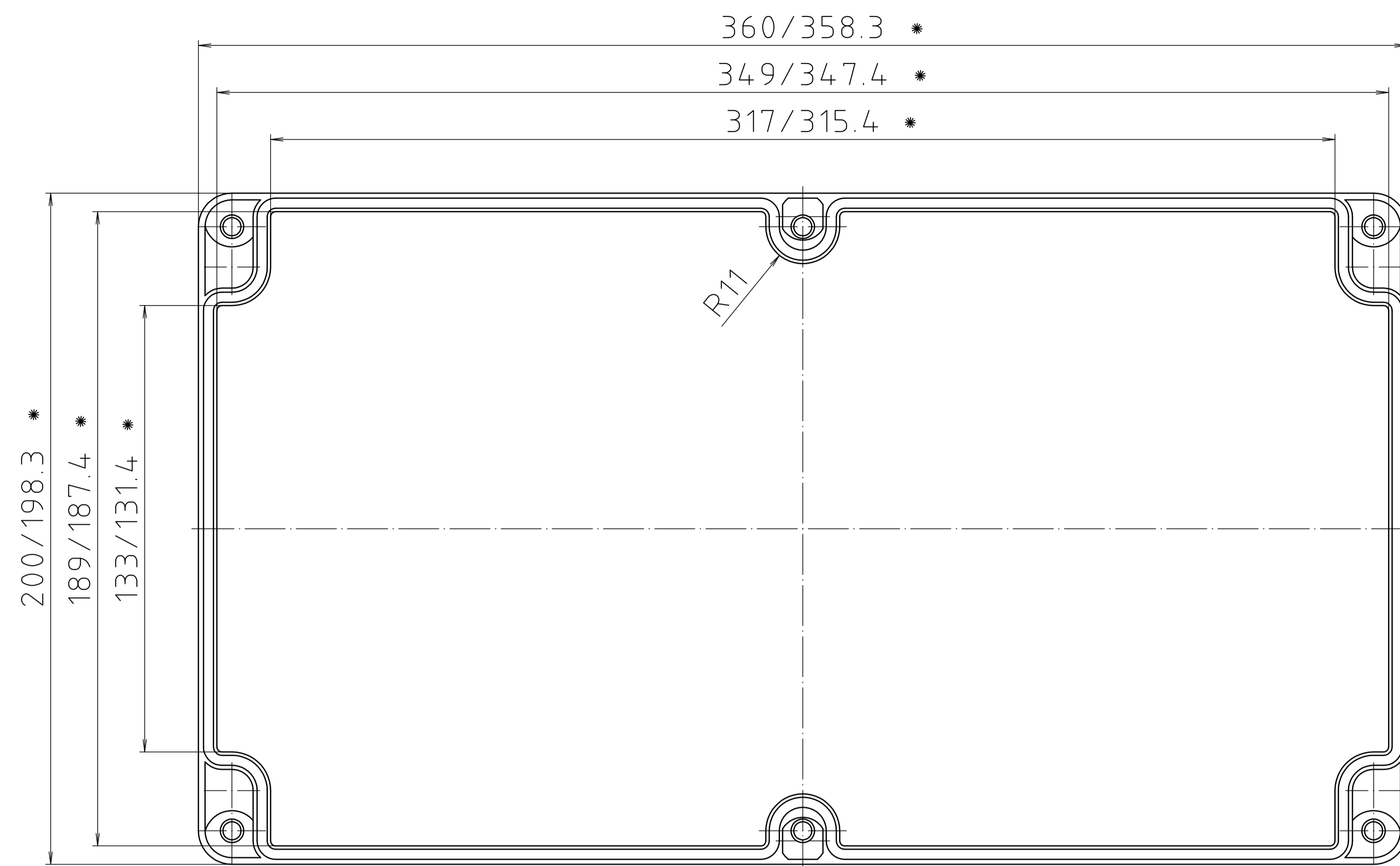
Deckel / lid
