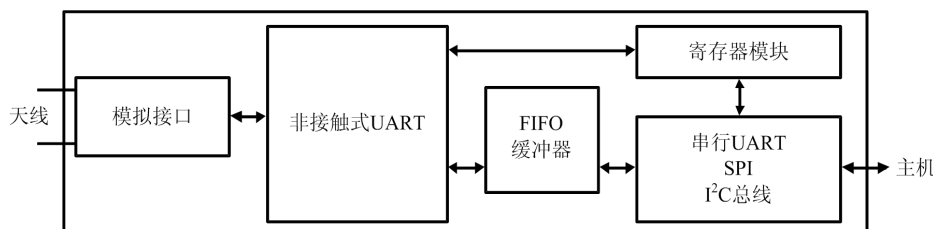
图 2.简化的 MS512 框图
