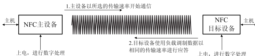
图 11. 被动式通信模式
