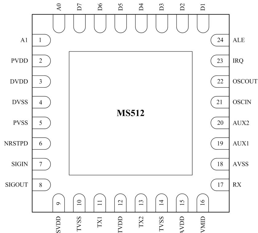
图 3. QFN32 封装
