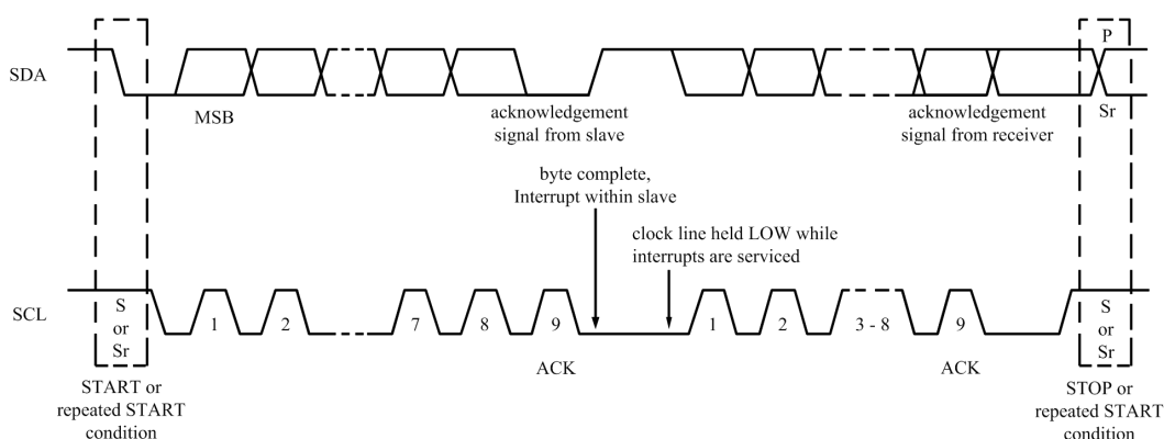
图 20. I 2 C 总线的数据传输
