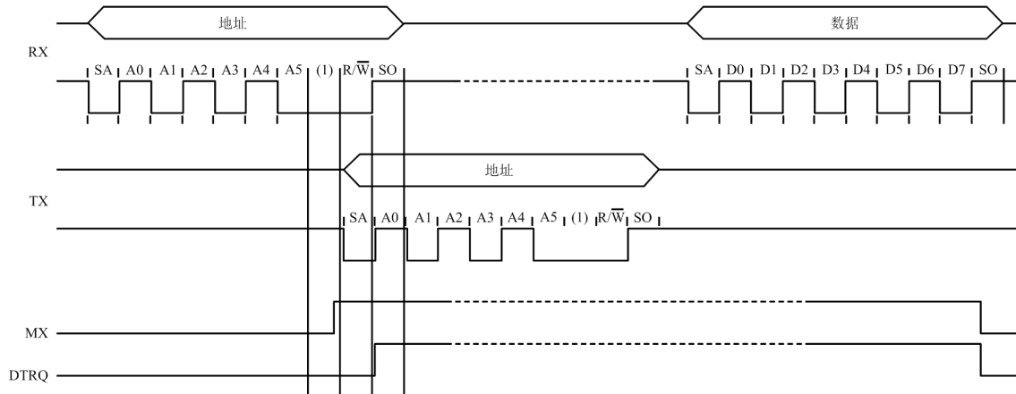
图 15. UART 写数据时序图
