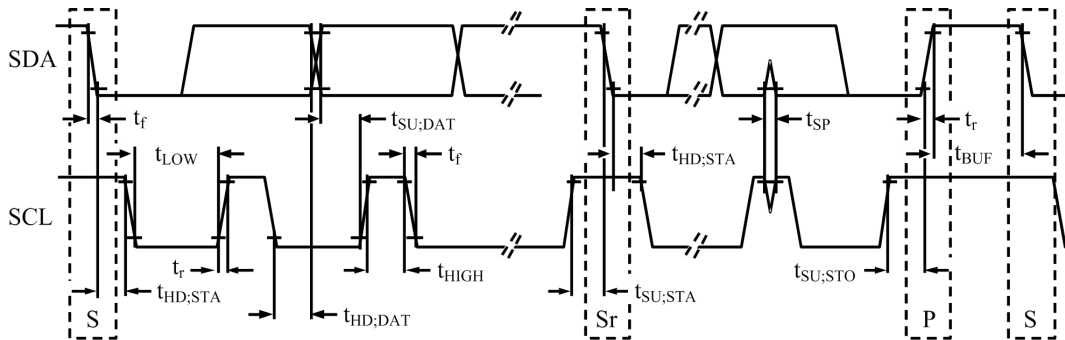
图 39. I 2 C 总线上快速和标准模式器件的时序
