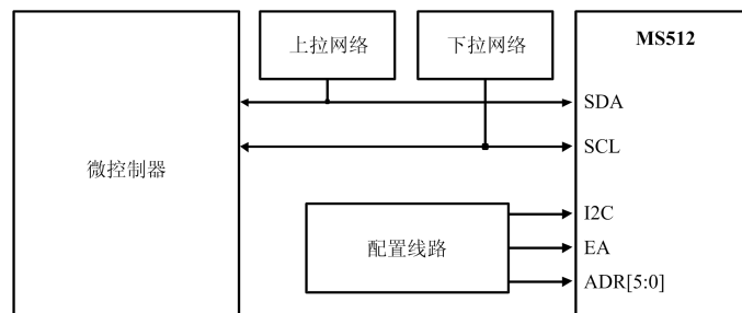
图 16. I 2 C 总线接口
