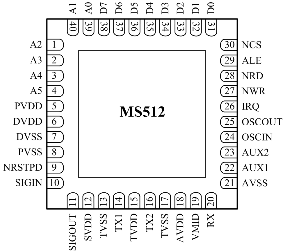
图 4. QFN40 封装
