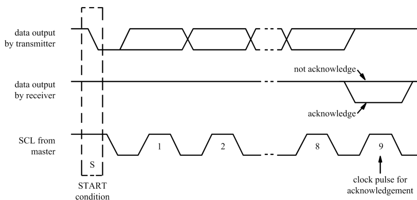
图 19. I 2 C 总线的应答
