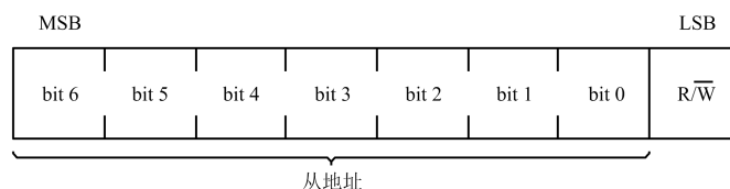
图 21. 起始条件后的第一个字节
