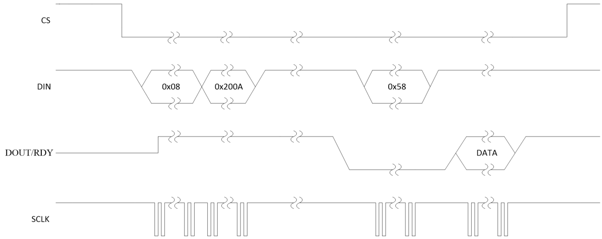
单次转换
