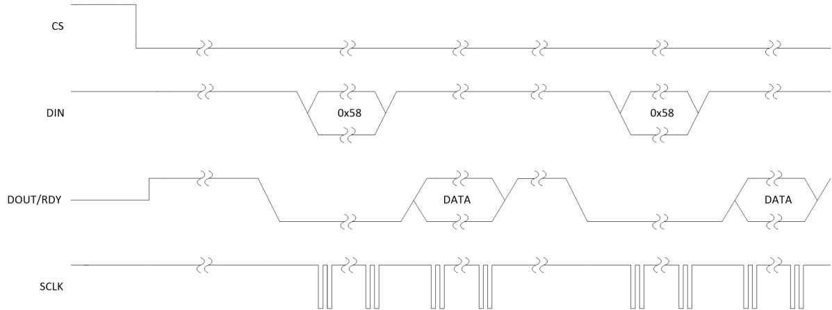
连续转换
