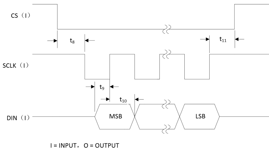
写入时序图
