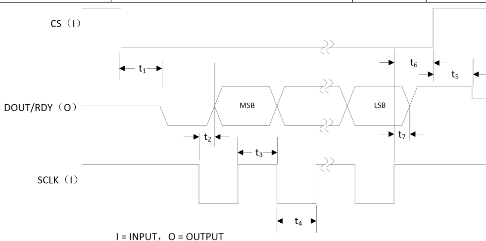
读取时序图
