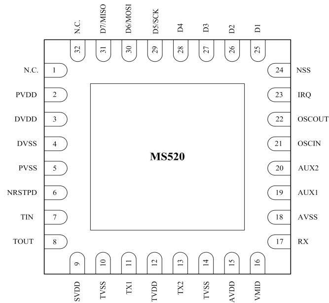
图 3. 封装
