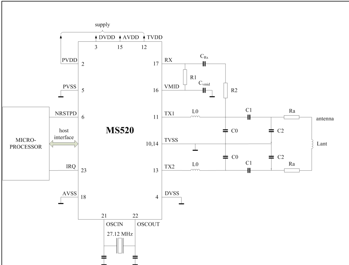
图 15. 典型应用图
